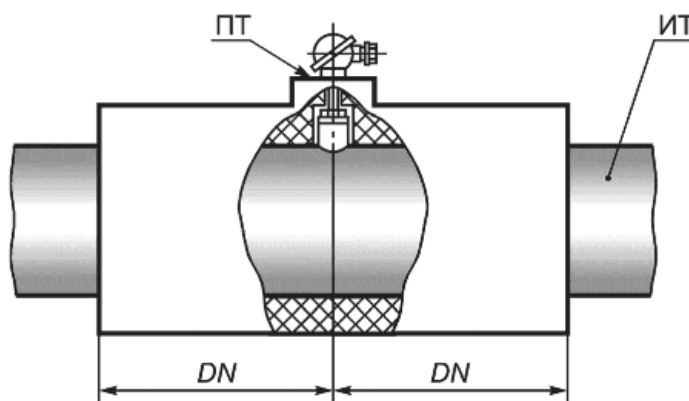
Рисунок 5 - Пример теплоизоляции участков ИТ и ПТ
